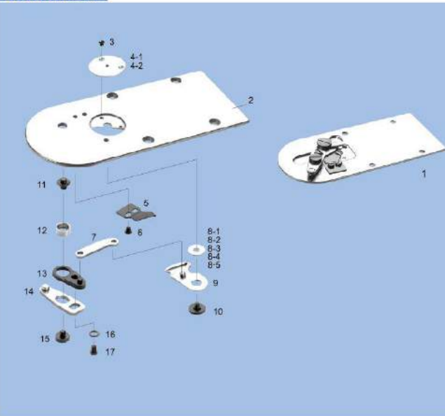
LK-1910/1920 剪线组件 ASSEMBLY FOR LK-1910/1920
