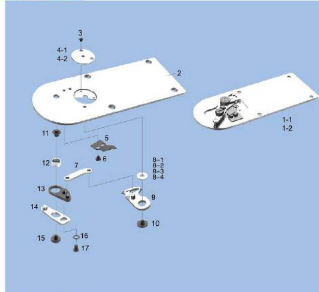
AMS-210D 剪线组件 ASSEMBLY FOR AMS-210D
