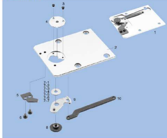
MOL-254后剪线组件 ASSEMBLY FOR MOL-254
