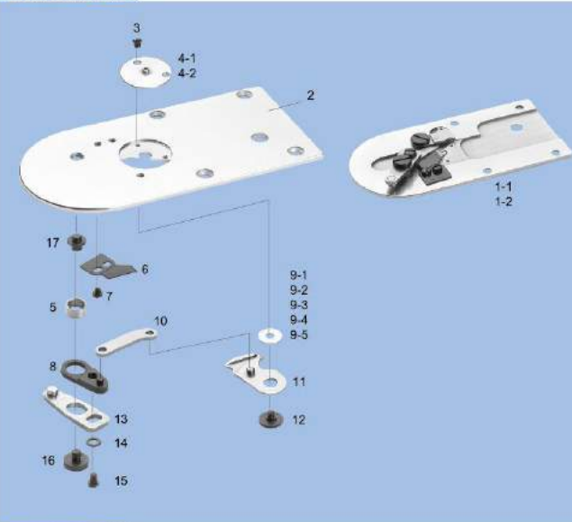
LK-1903A 剪线组件 ASSEMBLY FOR LK-1903A
