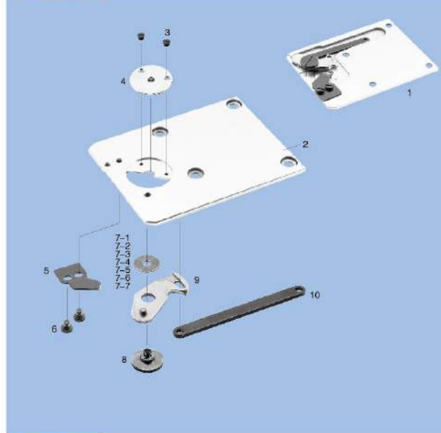
MOL-254前剪线组件 ASSEMBLY FOR MOL-254
