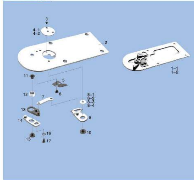
AMS-210E 剪线组件 ASSEMBLY FOR AMS-210E
