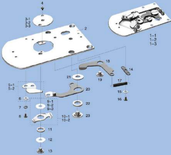
KE-430D 剪线组件 ASSEMBLY FOR KE-430D
